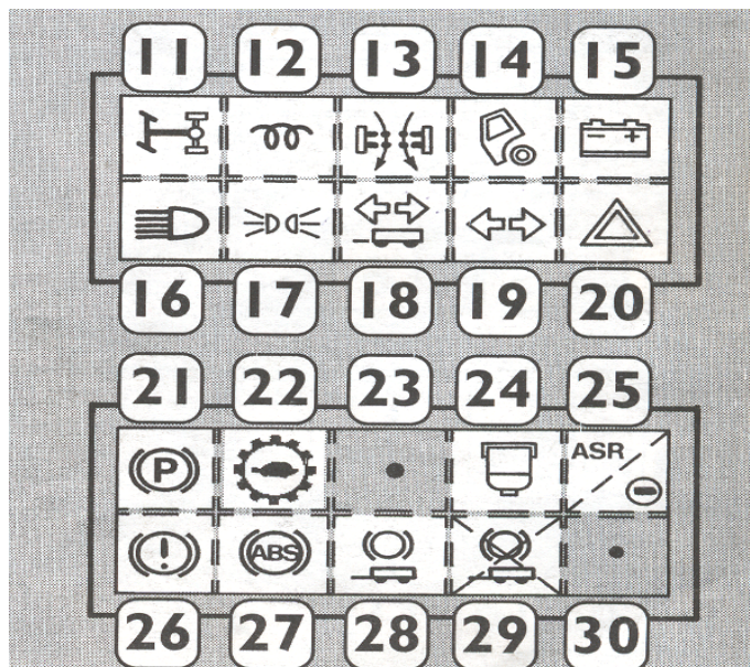
Abbildung der Anzeigen für Fahrerhausverriegelung, ABS, ASR, ...
